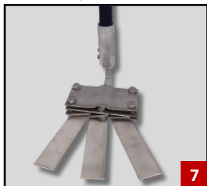
RACORD INOX PRIZĂ DE PĂMÂNT Exemplu de instalare
